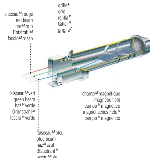
canon M à électrons M electron gun cañón M de electrones M Elektronenkanone F cannone M elettronico
